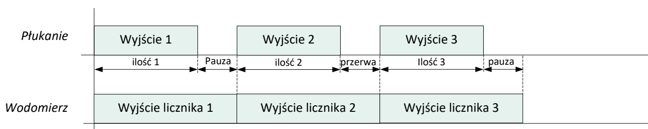
Rys.5 Płukanie na podstawie ilości
