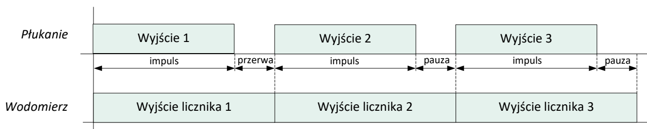
Rys.4 Płukanie na podstawie impulsu
