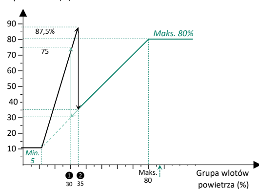
Wlot powietrza 1 (%)
