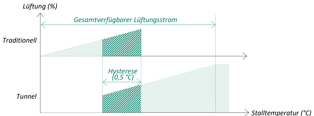
Traditionelle Lüftung
