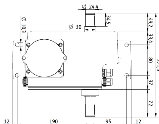
Afmetingen ELM-100-2A / ELM-250-2A
